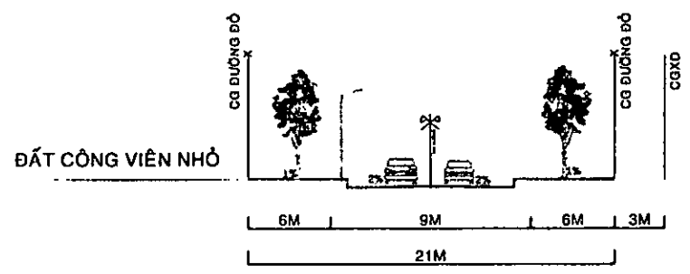
MẶT CẮT 8-8: ĐƯỜNG CÓ LỘ GIỚI 21M
