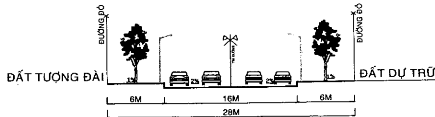
MẶT CẮT 3'-3': ĐƯỜNG CÓ LỘ GIỚI 28M
