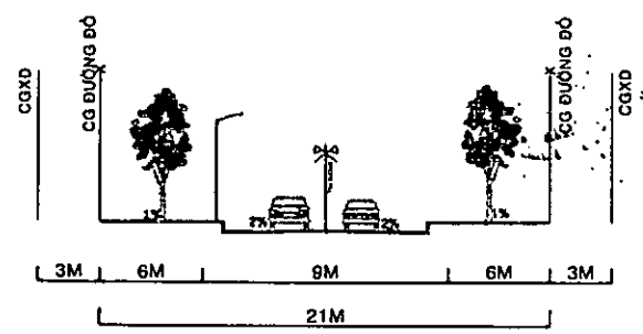
MẶT CẮT 6-6: ĐƯỜNG CÓ LỘ GIỚI 21M
